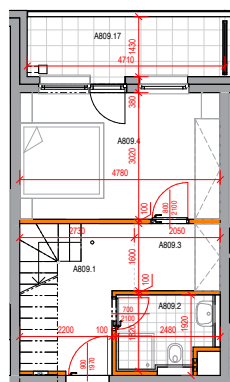
A809_8np M 1 : 75
