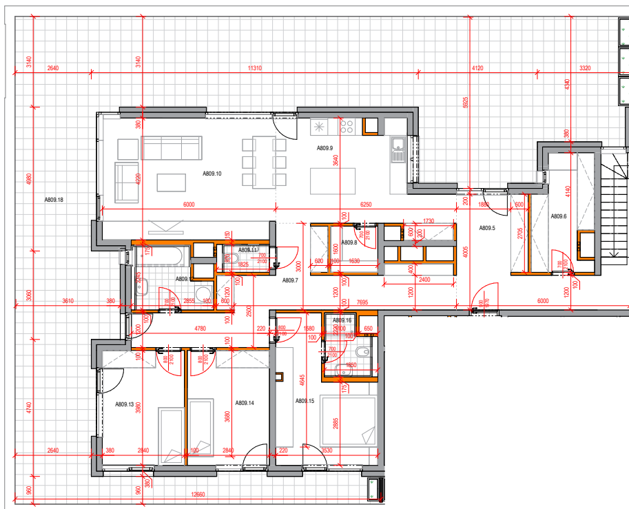
A809_9np M 1 : 75
